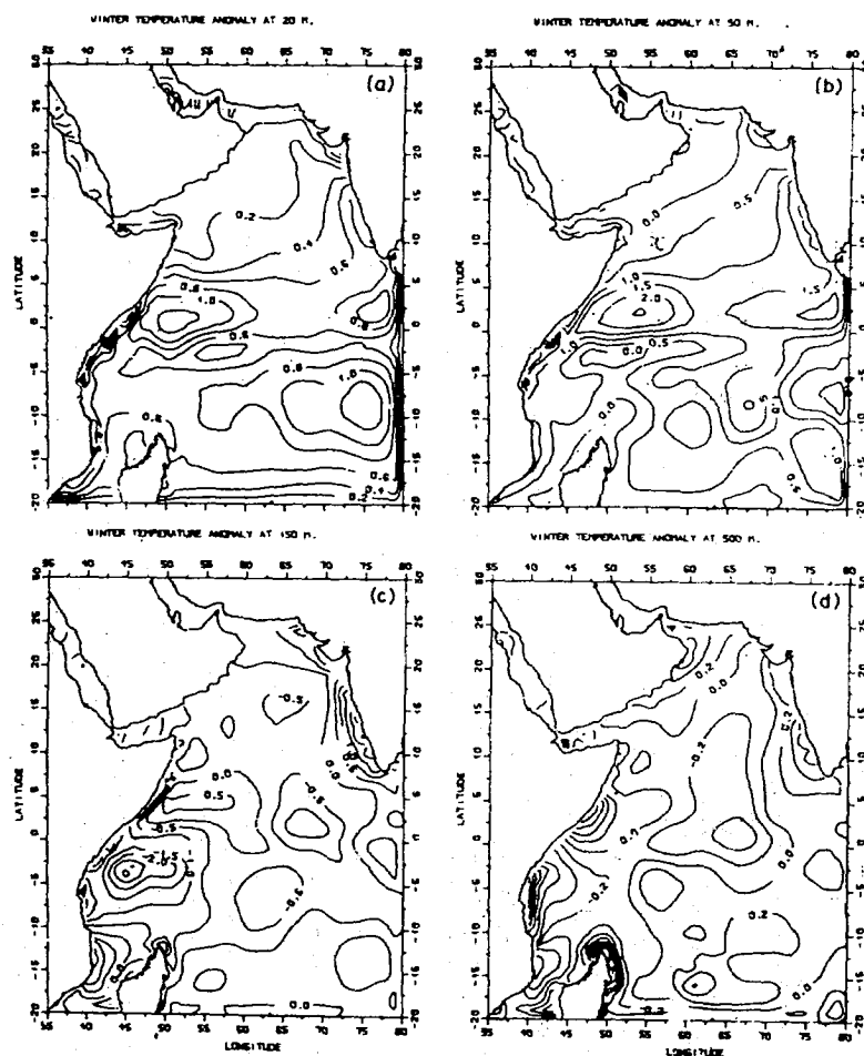
Fig. 6—Temperature anomaly fields at (a) 20 m (b) 50 m (c) 150 m (d) 300 m depths.
